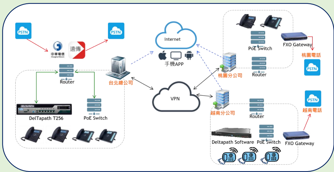
▲ 易通科技協助客戶建置 Deltapath 整合通訊解決方案之架構圖
